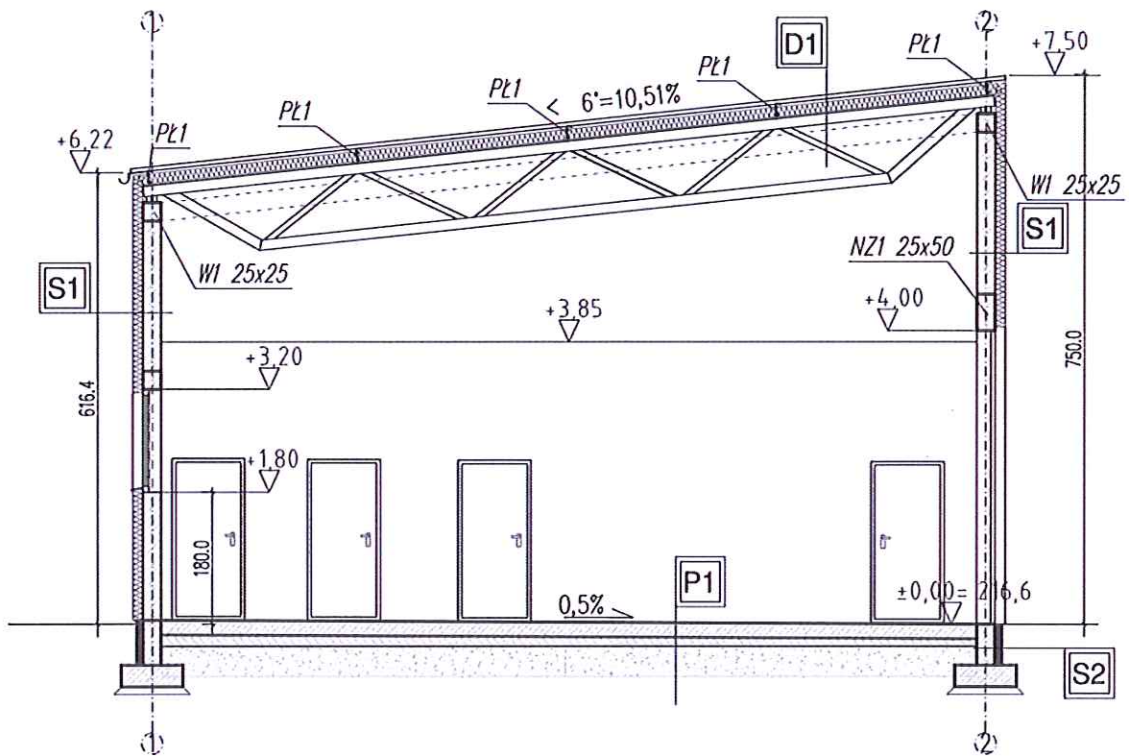
HALA WARSZTATOWO-MAGAZYNOWA - PRZEKRÓJ A-A
