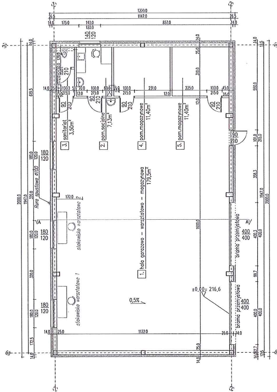
HALA WARSZTATOWO-MAGAZYNOWA - RZUT PRZYZIEMIA
